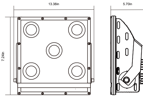
FL-3150
