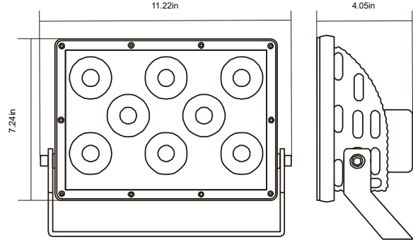
FL-3060
