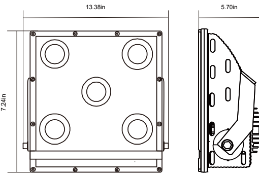
FL-3100
