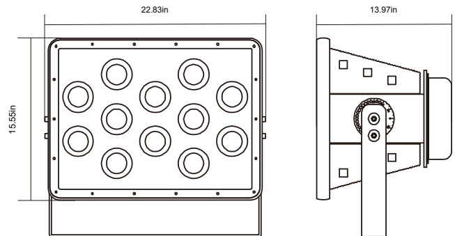
FL-3520
