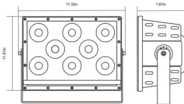
FL-3250
